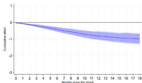
(e) El Niño. Food inflation (BU)
