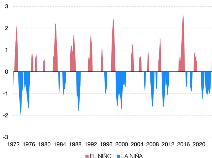
Figure 2: Episodes of El Niño and La Niña
