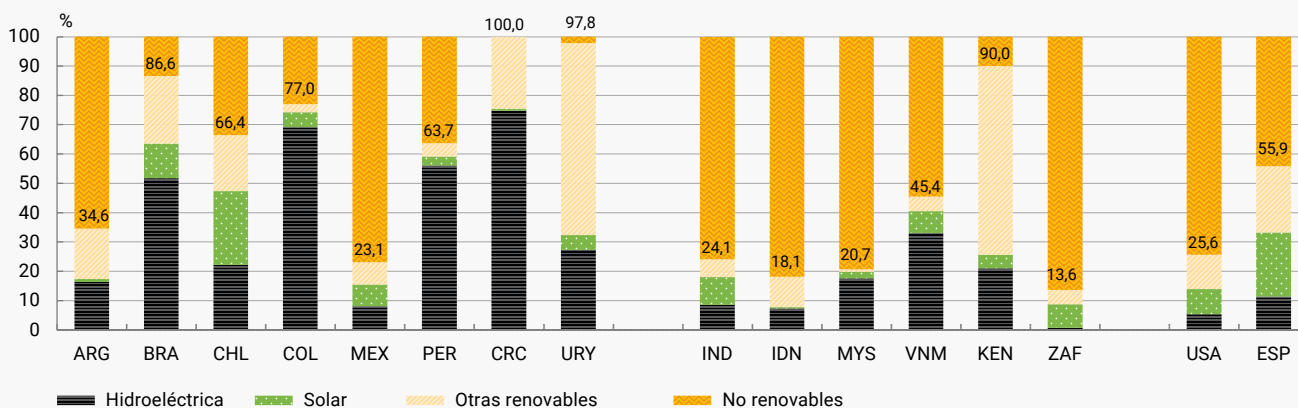
Gráfico 1 Composición de la matriz de generación de energía eléctrica (2025)
