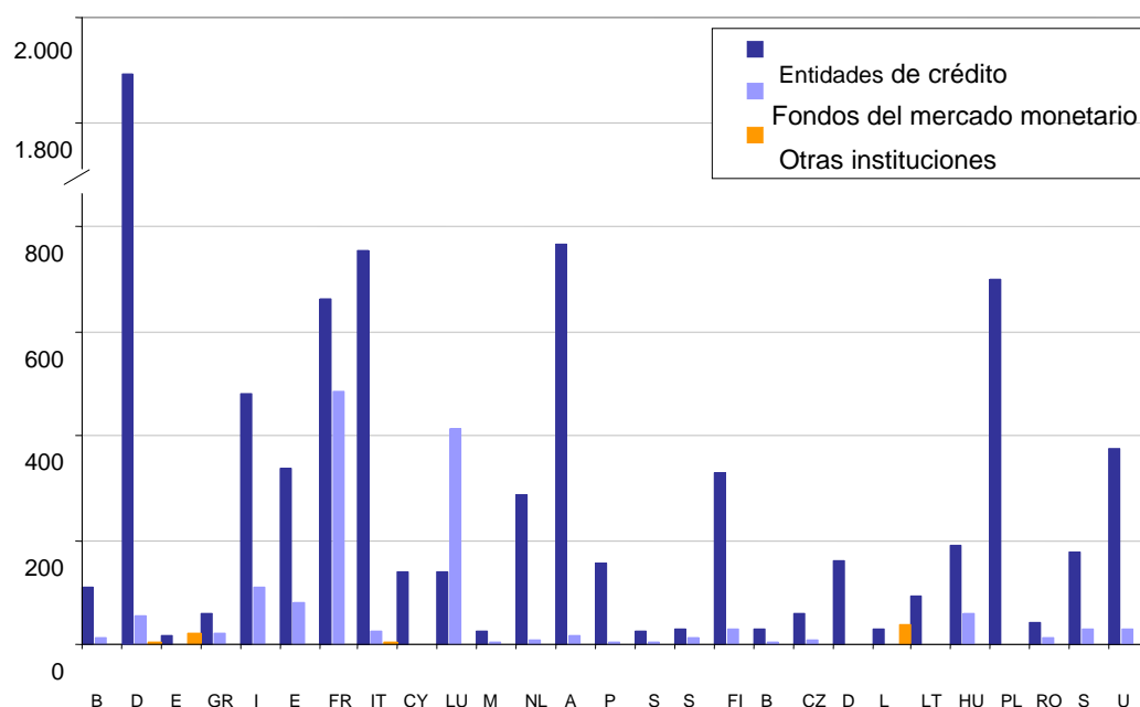
Gráfico 2 – Número de IFM (excluidos los bancos centrales y el Banco Europeo de Inversiones) en la UE, por países y categoría (a 1 de enero de 2012)
