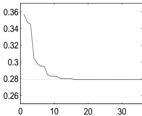
a) SA series
